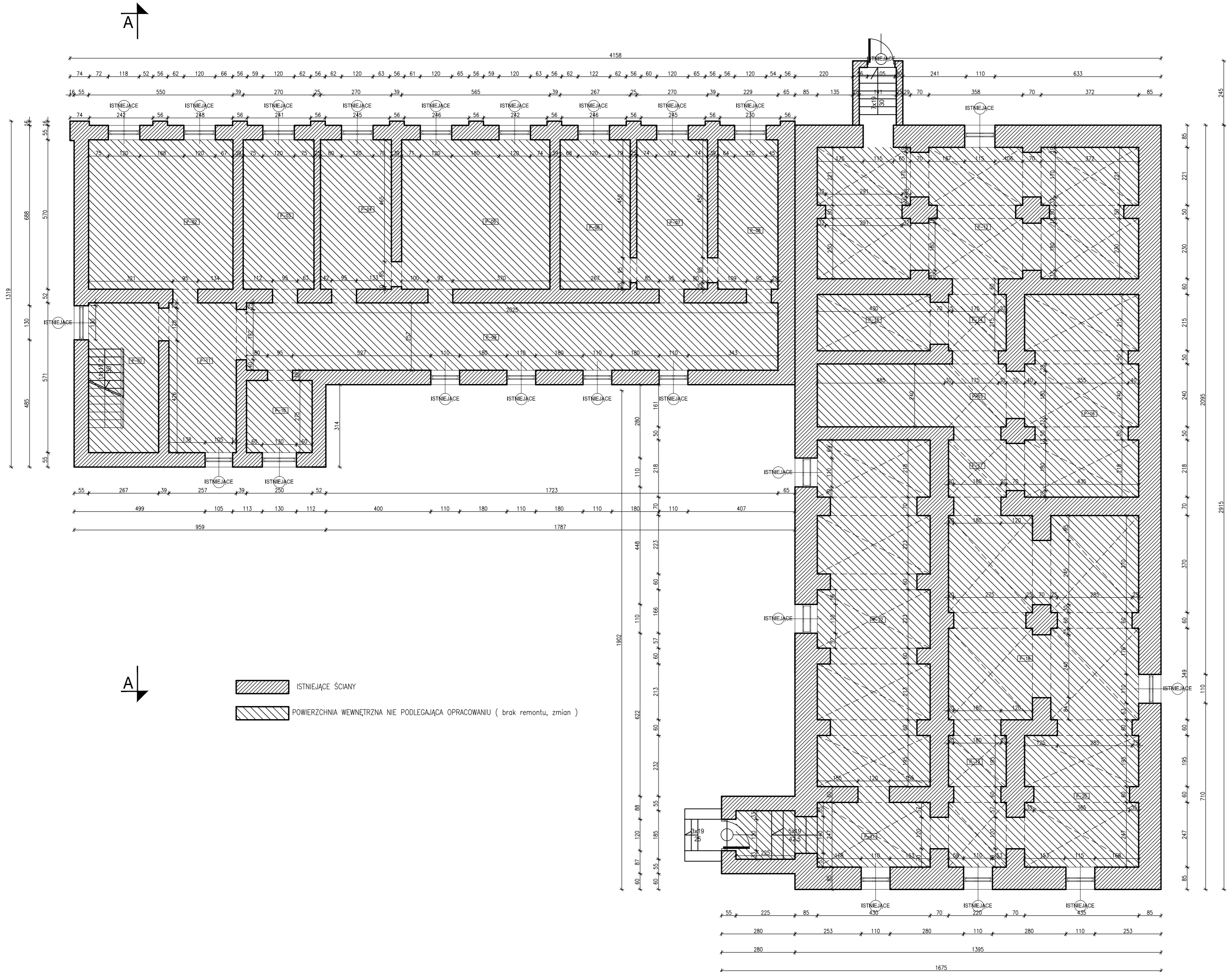
WYKAZ POWIERZCHNI – PIWNICA
