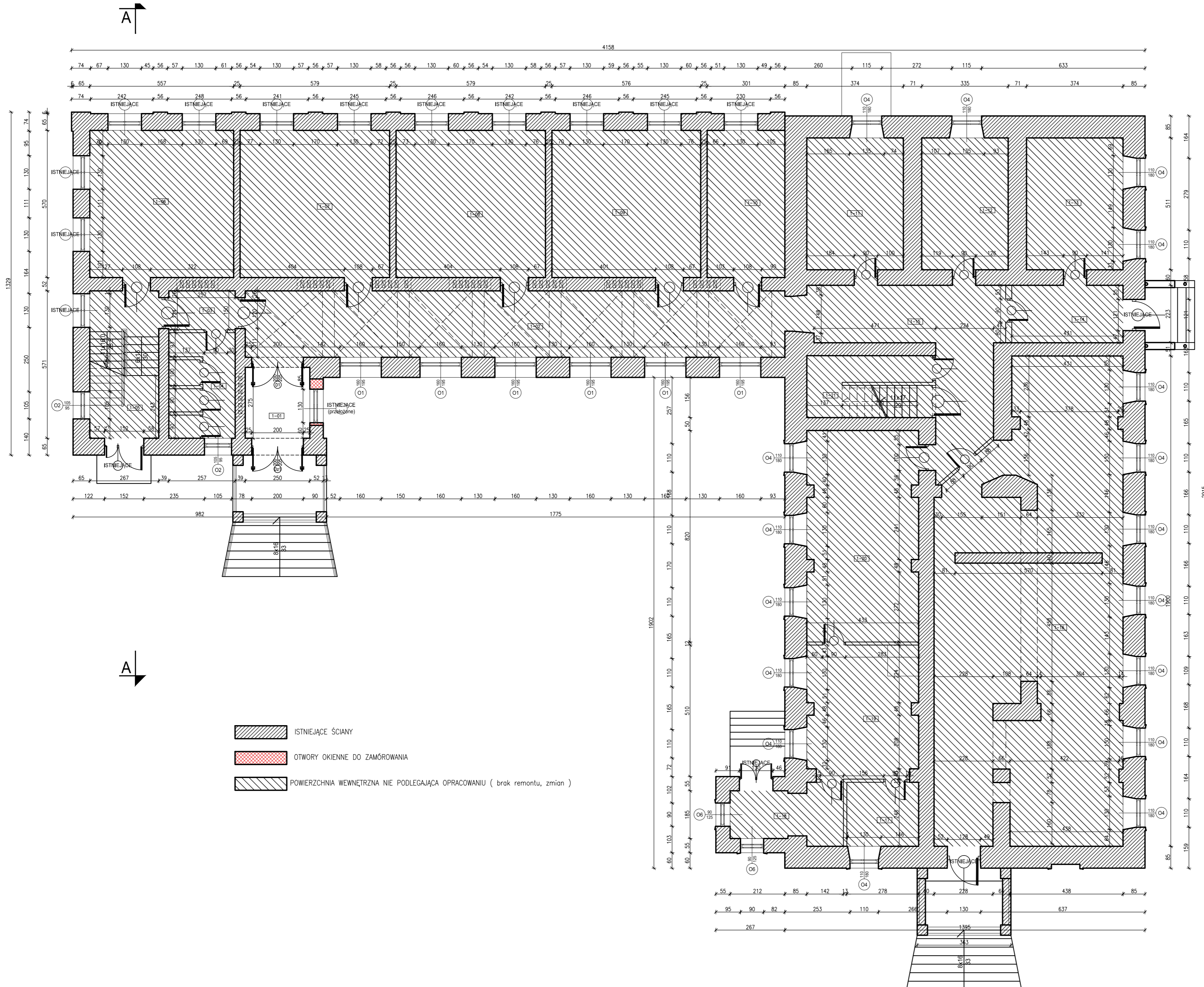
WYKAZ POWIERZCHNI – PARTER
